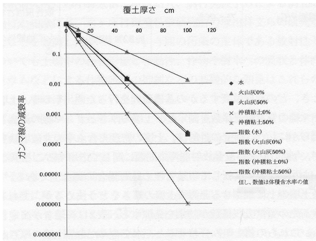
図1 覆土厚さと減衰率の予測[5]
