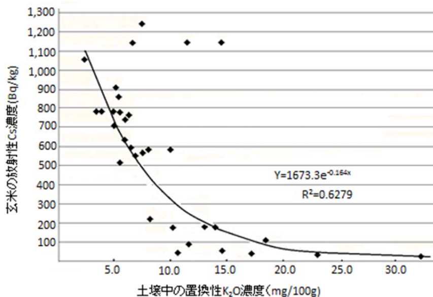
図2 土壌中の置換性カリウム濃度と玄米の放射性セシウム濃度との関係[13]
