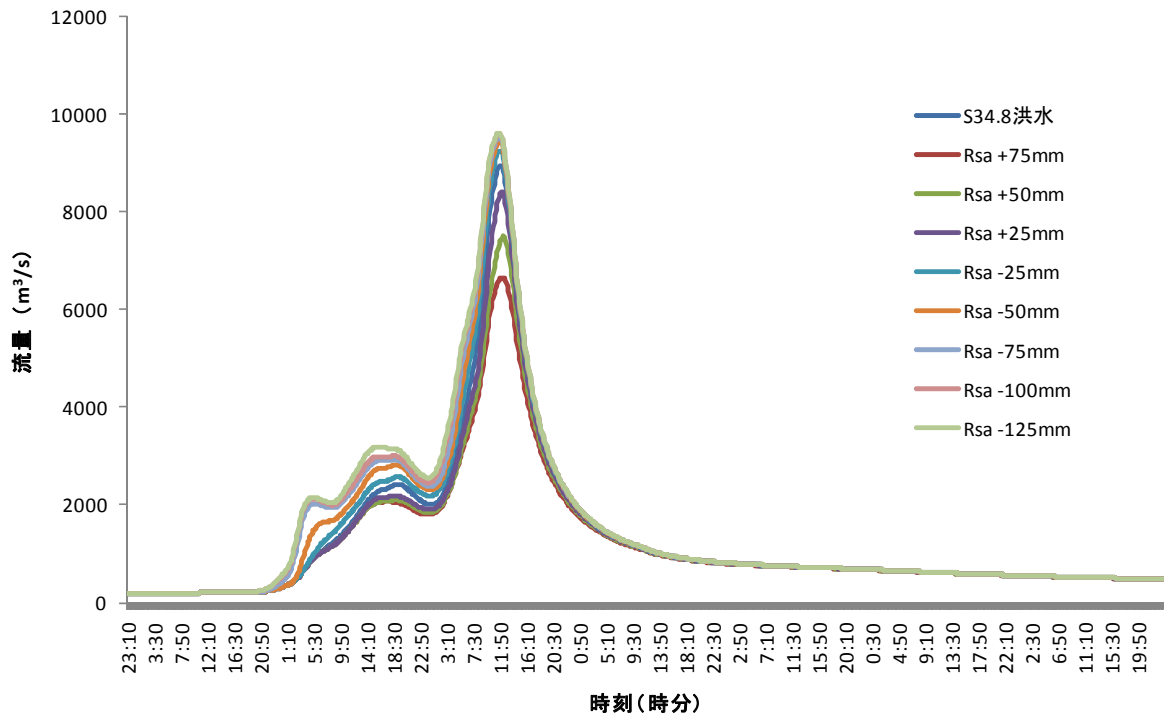
図18：Rsaの値が昭和34年8月洪水の八斗島地点での計算結果に与える影響
