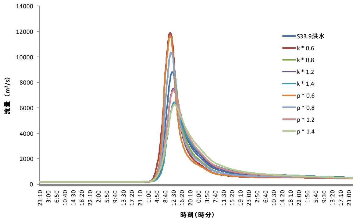
図 2 1 : k, p の値が昭和 33 年 9 月洪水の八斗島地点での計算結果に与える影響
