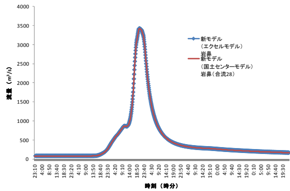
図10：岩鼻地点（烏川流域）
