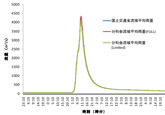
図 3 8 : 岩鼻地点 (烏川流域)
