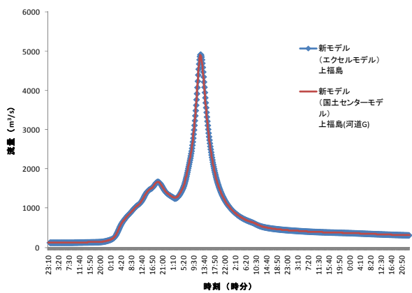
図5：上福島地点（吾妻川流域）
