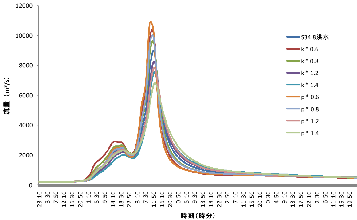
図22：k, pの値が昭和34年8月洪水の八斗島地点での計算結果に与える影響
