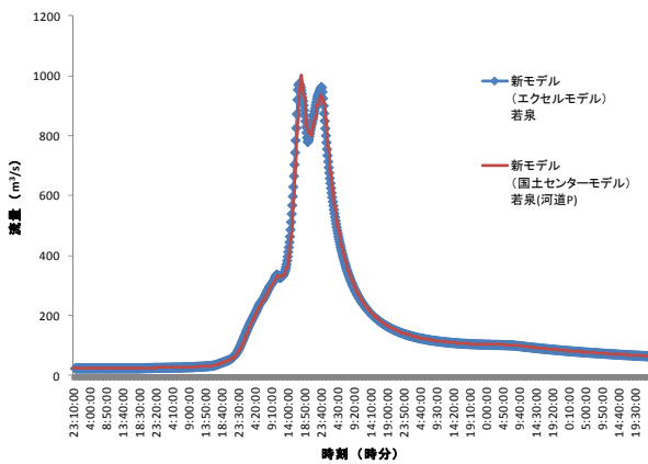
図11：若泉地点（神流川流域）
