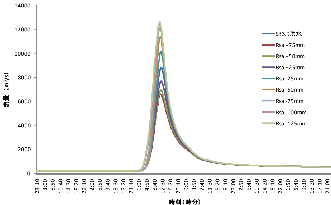
図17：Rsaの値が昭和33年9月洪水の八斗島地点での計算結果に与える影響
