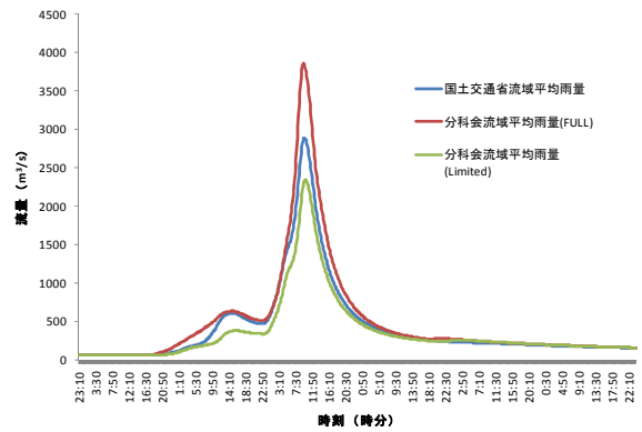
図30：岩鼻地点（烏川流域）
