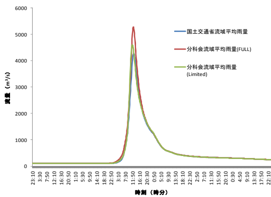
図 25：上福島地点（吾妻川流域）
