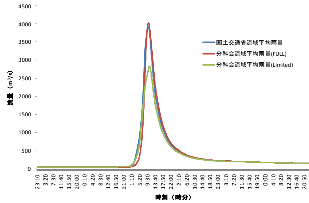
図 26：岩鼻地点（烏川流域）
