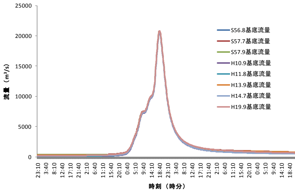
図 4 1 : 新モデルによる昭和 22 年 9 月洪水の再現計算結果
