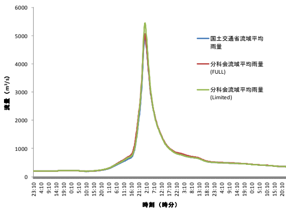
図33：上福島地点（吾妻川流域）
