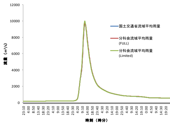
図 4 0 : 八斗島地点 (利根川流域)
