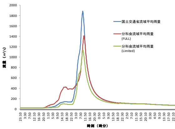
図31：若泉地点（神流川流域）
