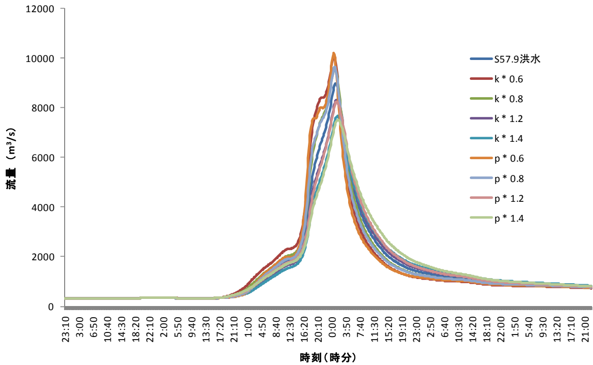
図23 : k, p の値が昭和57年9月洪水の八斗島地点での計算結果に与える影響
