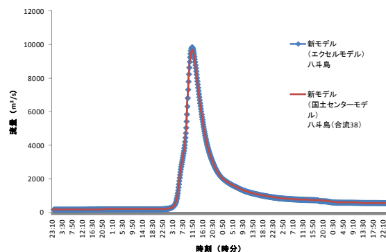
図16：八斗島地点（利根川流域）
