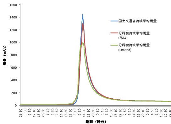
図 27：若泉地点（神流川流域）
