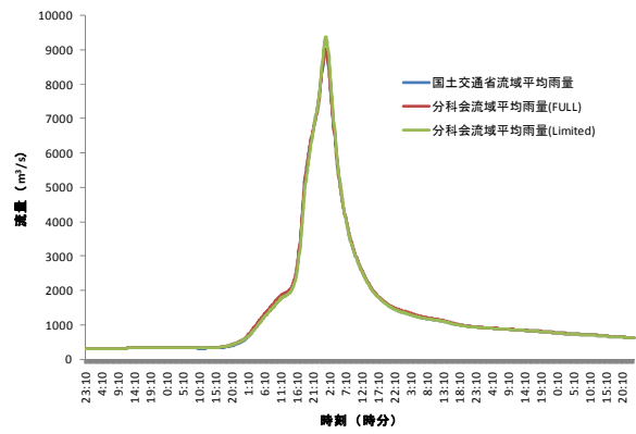
図 3 6 : 八斗島地点 (利根川流域)
