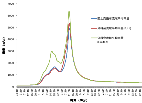
図29：上福島地点（吾妻川流域）
