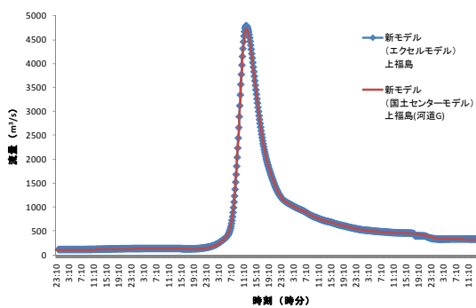
図13：上福島地点（吾妻川流域）
