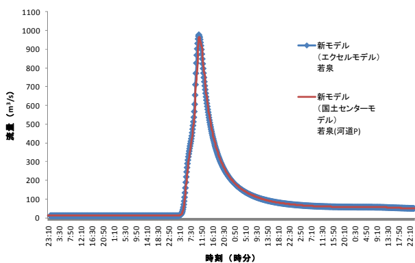
図15：若泉地点（神流川流域）
