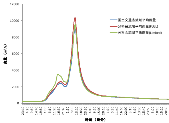
図32：八斗島地点（利根川流域）
