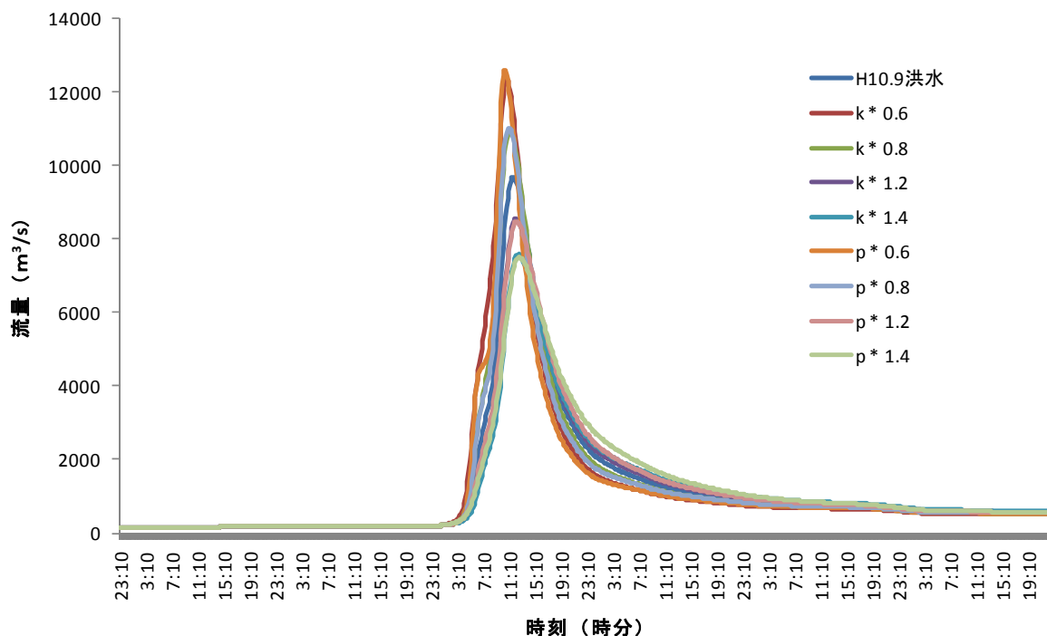
図24：k, p の値が平成10年9月洪水の八斗島地点での計算結果に与える影響
