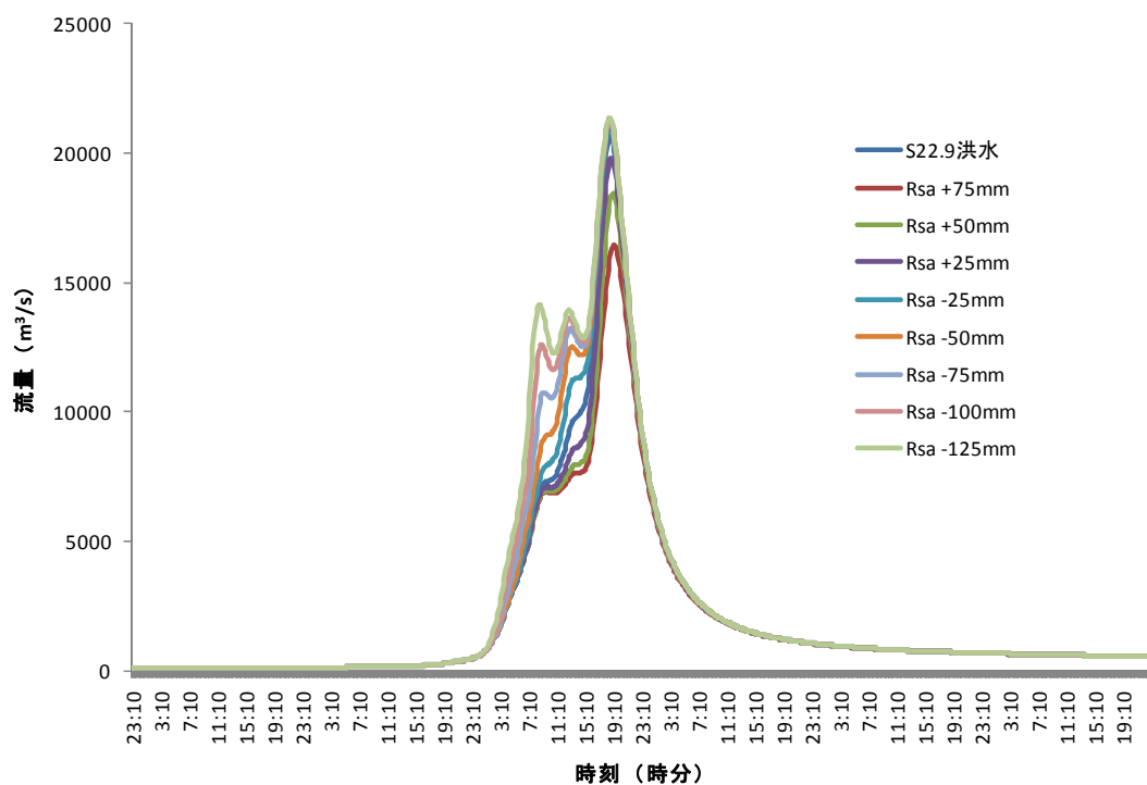
図42: R_{sa} の値が昭和22年9月洪水の再現結果に与える影響
