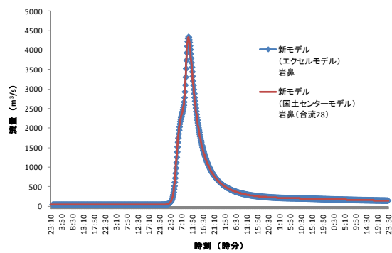
図14：岩鼻地点（烏川流域）
