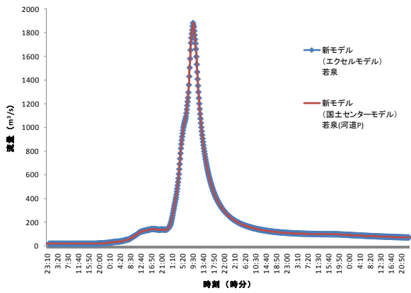
図7：若泉地点（神流川流域）
