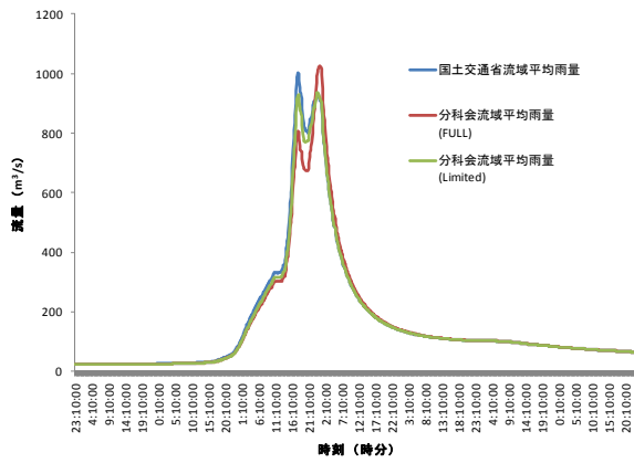
図 3 5 : 若泉地点 (神流川流域)
