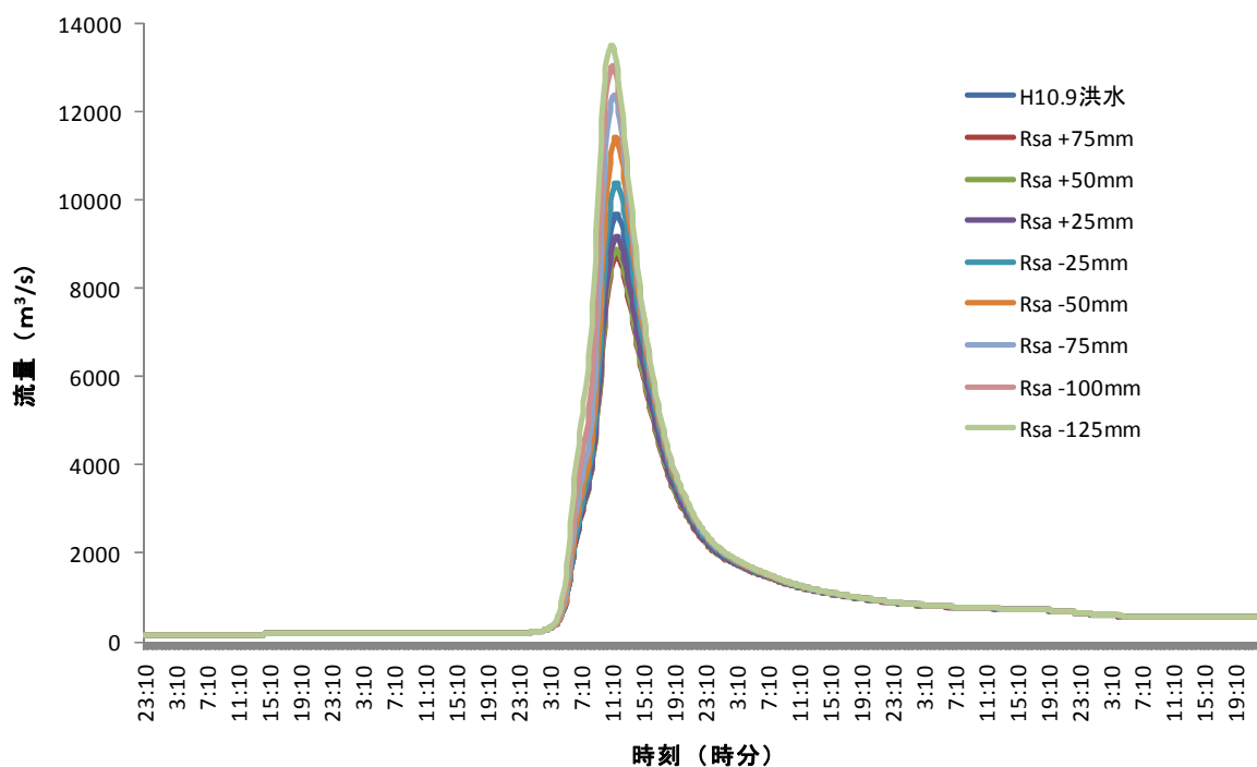
図20：Rsaの値が平成10年9月洪水の八斗島地点での計算結果に与える影響
