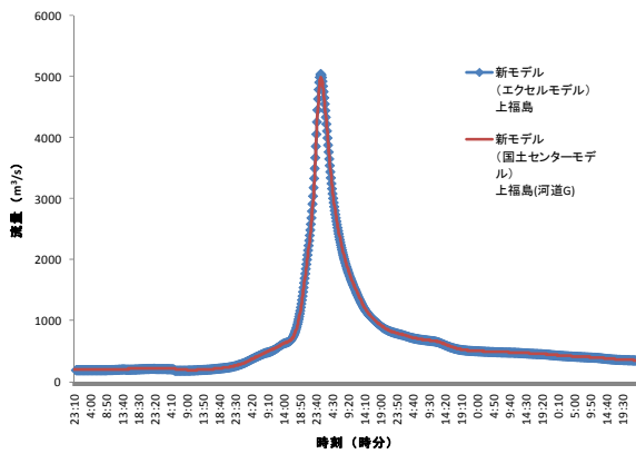
図9：上福島地点（吾妻川流域）
