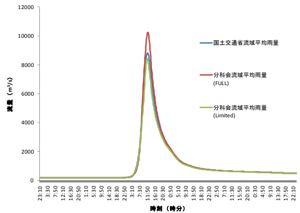
図 28：八斗島地点（利根川流域）
