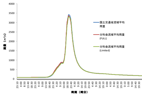
図34：岩鼻地点（烏川流域）
