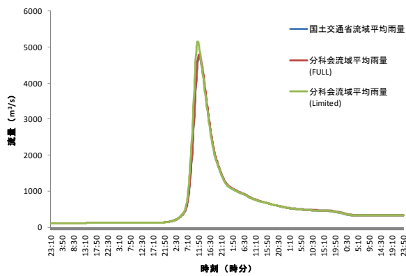
図 3 7 : 上福島地点 (吾妻川流域)
