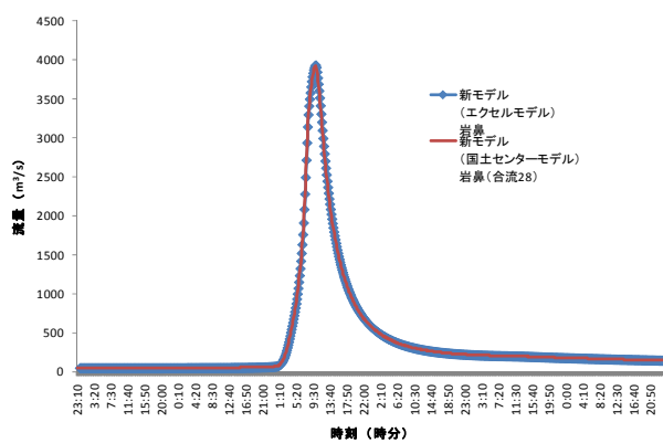
図2：岩鼻地点（烏川流域）
