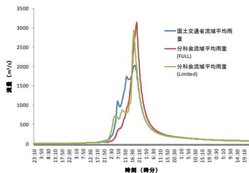
図 4 5 : 若泉地点 (神流川流域)
