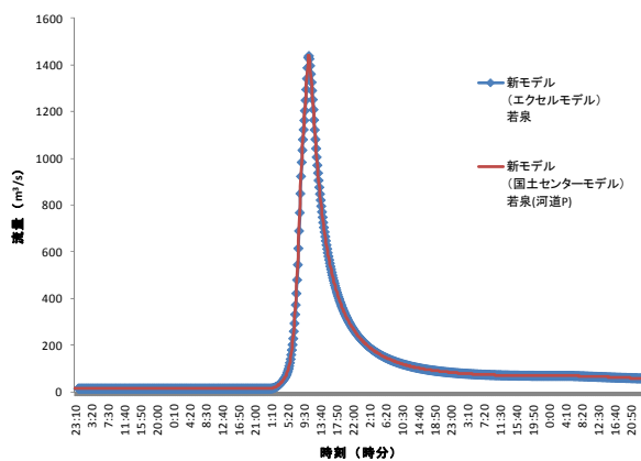
図3：若泉地点（神流川流域）
