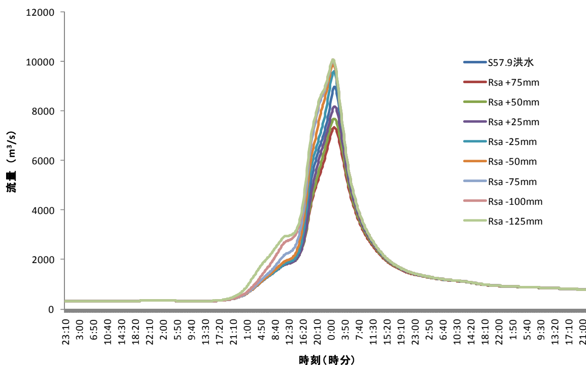
図19：Rsaの値が昭和57年9月洪水の八斗島地点での計算結果に与える影響
