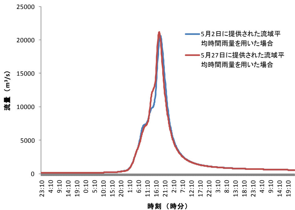
図 4 7 : 新たに推定された流域平均雨量を用いた昭和 22 年 9 月洪水の再現計算結果
