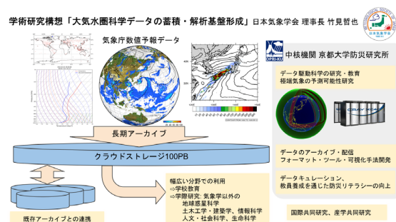
図2 大気水圏科学のデータの蓄積・解析基盤形成
