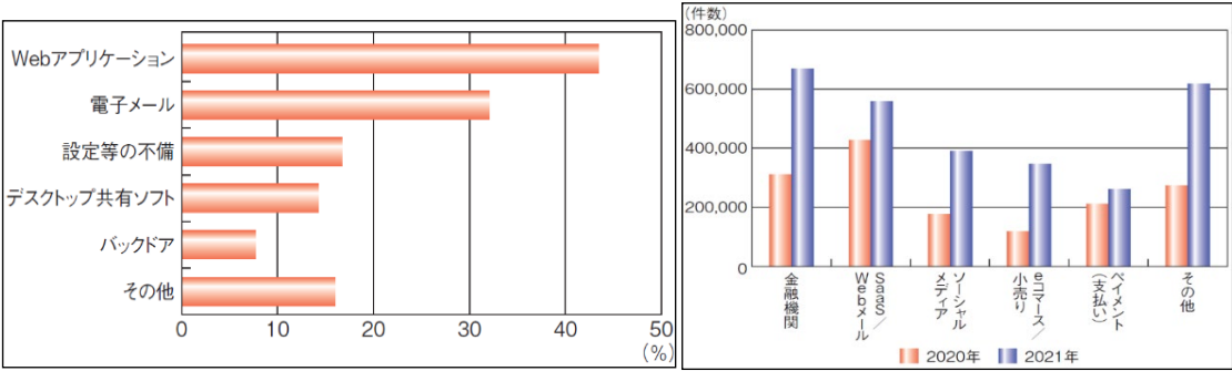
図 2.1.1 情報漏洩／侵害の侵入手口 (2021 年, n=3,279) 図 2.1.2 業種別のフィッシングサイト件数 (2020 年と 2021 年の比較) (出典) 情報セキュリティ白書 2022 (出典) 情報セキュリティ白書 2022
