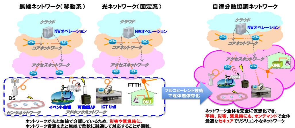
図6 サイバー・フィジカル空間を融合するための 光・無線融合型自律分散協調情報通信ネットワーク (出典) 第23期「学術の大型研究計画に関するマスタープラン」
