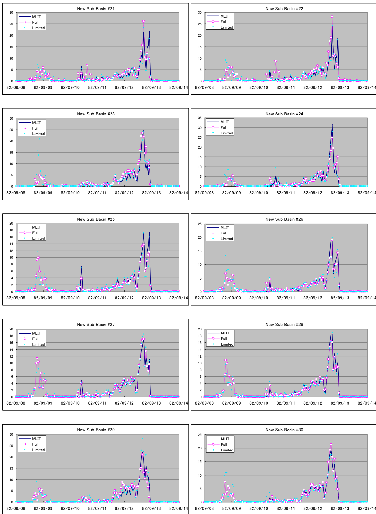
図 1d 新モデルサブ流域平均雨量（昭和 57 年年洪水）
