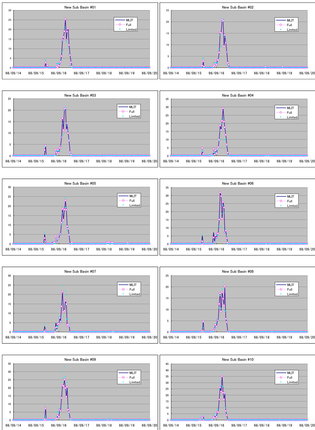
図 1e 新モデルサブ流域平均雨量 (平成 10 年年洪水)
