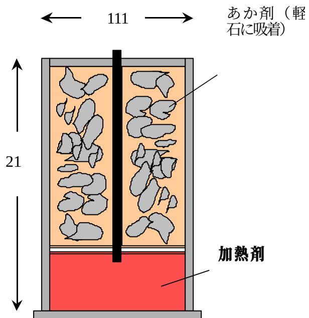
図 4 有毒発煙筒（あか筒）の構造
