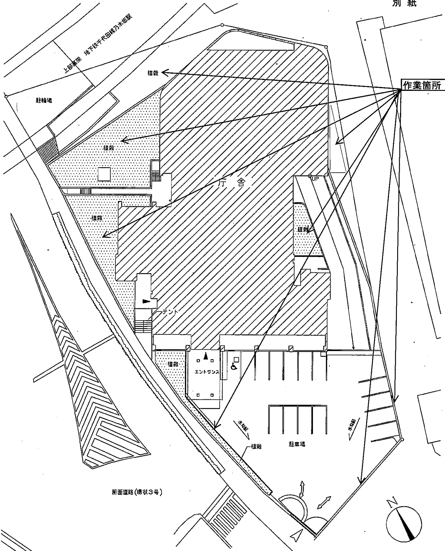
配置図 1/200
