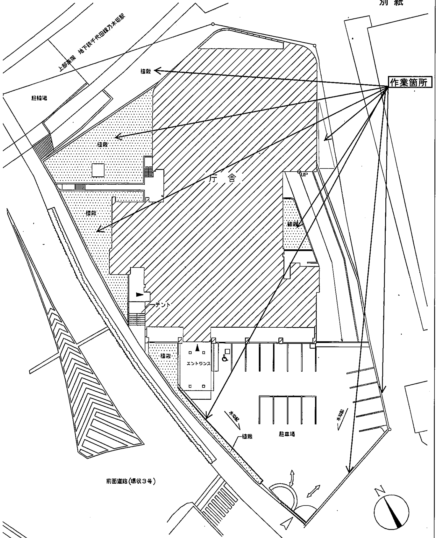
配置図 1/200
