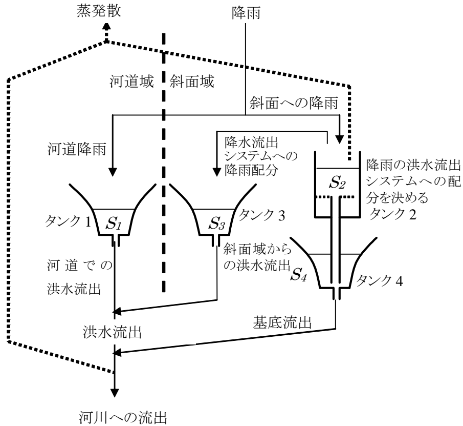
図8 HYCYMODEL の説明図
