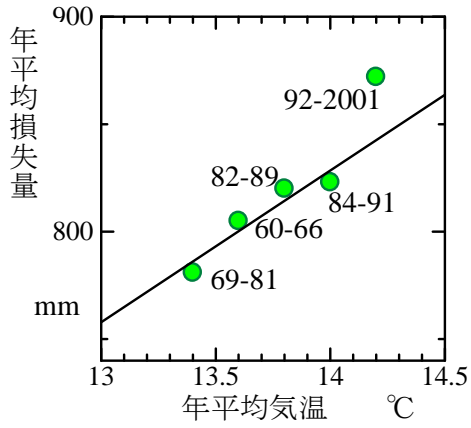
図5 竜ノ口山北谷における年末基底流出高が 相等しい期間における年平均損失量の 年平均気温に対する関係
