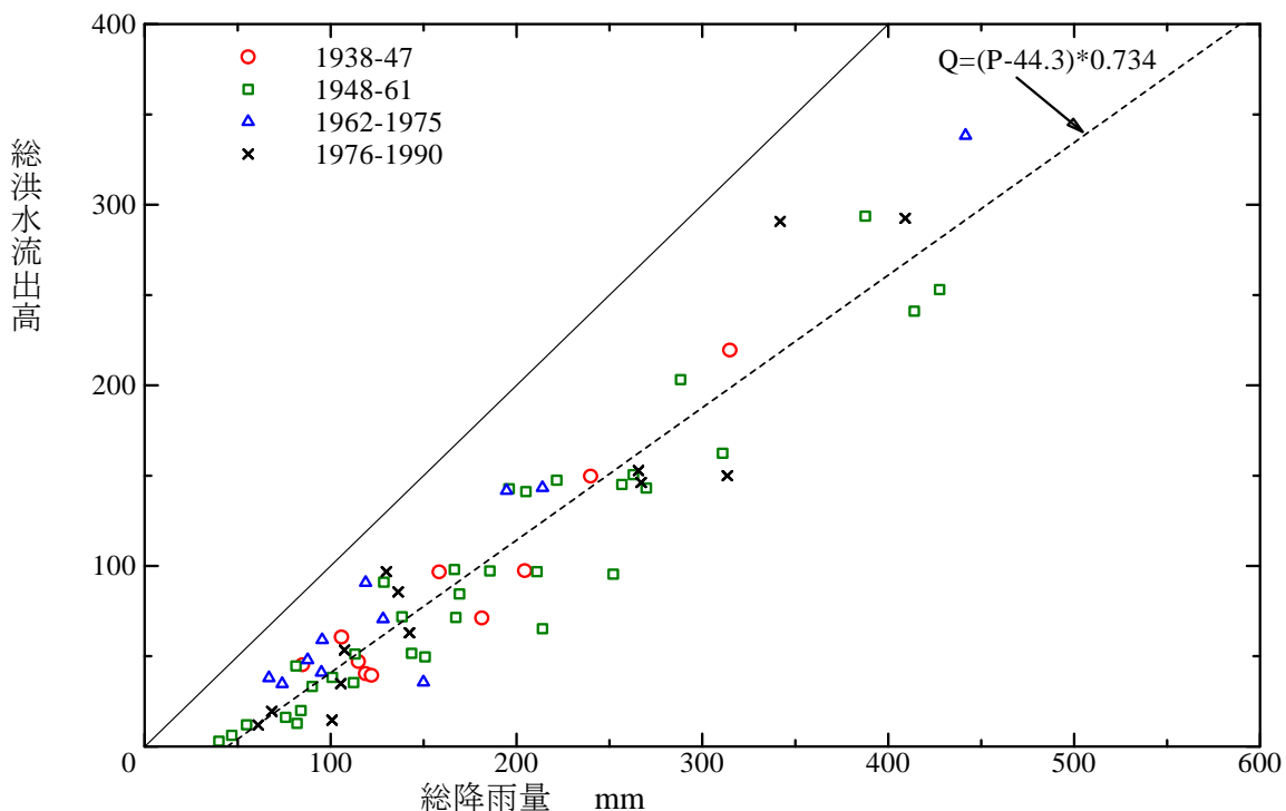
図3 宝川本流の1938～90年の出水における総降雨量と総洪水流出高の関係
