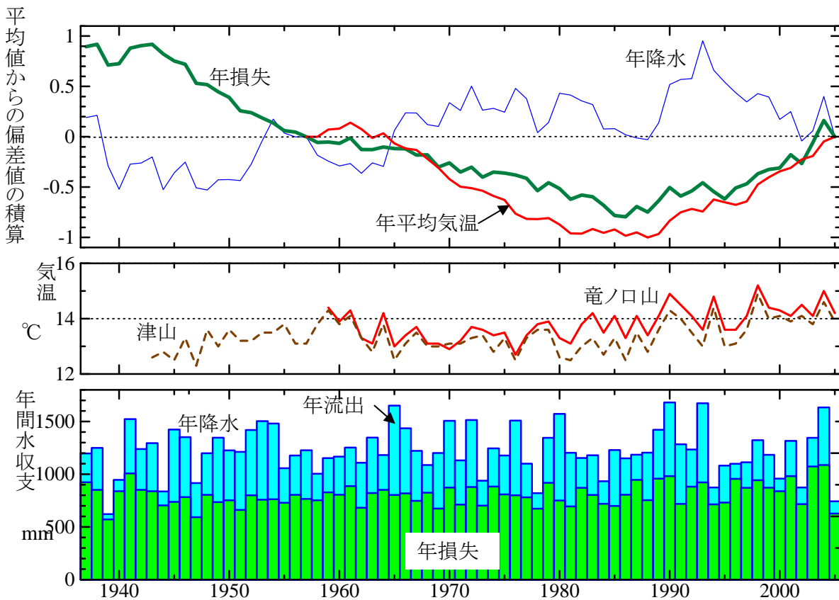
図4 竜ノ口山北谷における年間水収支(下段), 年平均気温(中段), 偏差積算曲線(上段)
