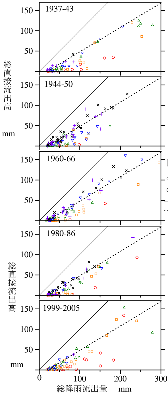
図7 竜ノ口山北谷の出水における5つの期間 毎の総降雨量と総洪水流出高の関係
