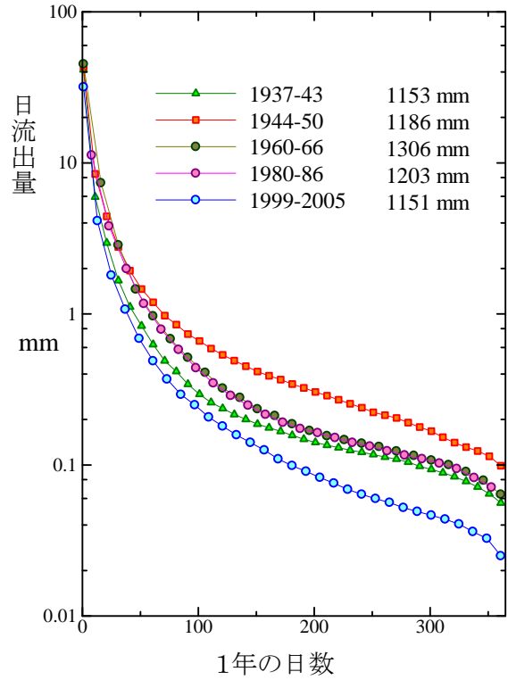
図6 竜ノ口山北谷の流況曲線 図中の数字は平均期間とその期 間の年平均降水量を示す
