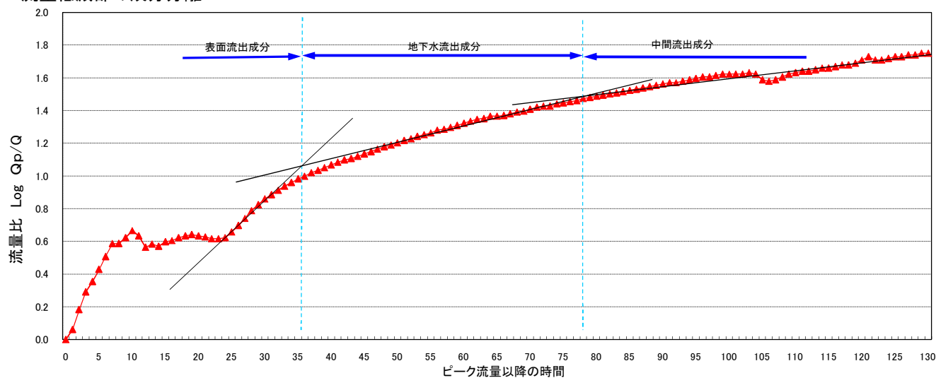
流量低減部の成分分離
