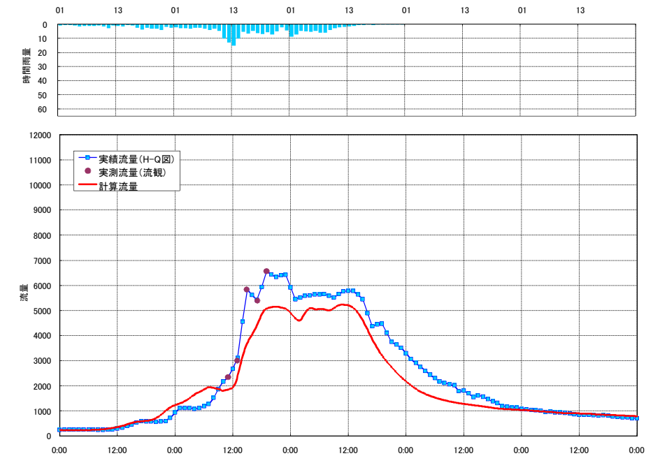
流出計算結果 平成13年9月洪水 八斗島 (利根川)
