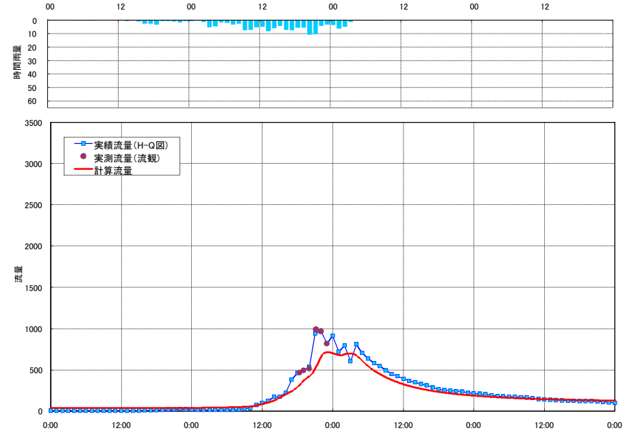
流出計算結果 平成14年7月洪水 村上 (吾妻川)
