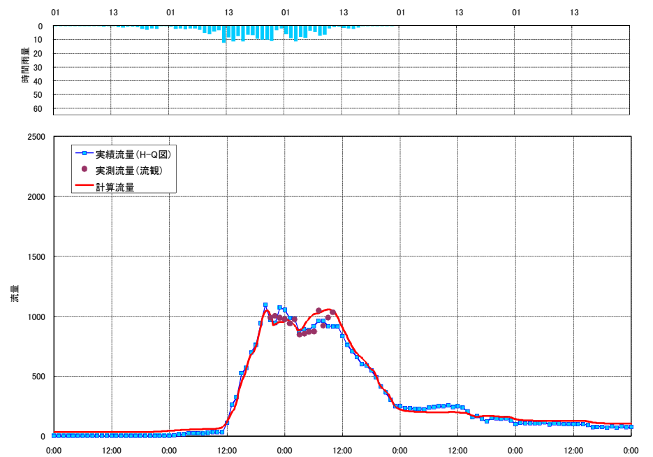
流出計算結果 平成13年9月洪水 上久屋 (片品川)
