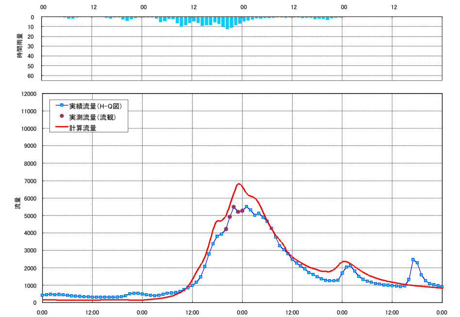
流出計算結果 平成11年8月洪水 八斗島 (利根川)
