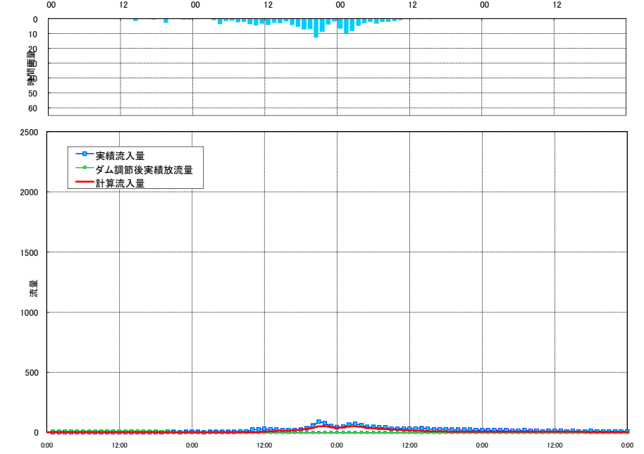
流出計算結果 平成14年7月洪水 相俣ダム (赤谷川)
