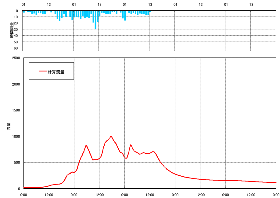
流出計算結果 平成13年9月洪水 若泉 (神流川)
