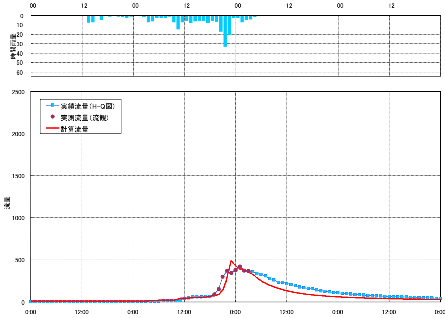
流出計算結果 平成14年7月洪水 藪原ダム (片品川)
