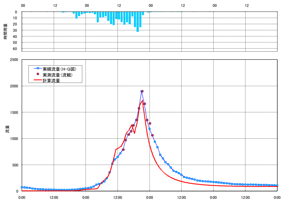
流出計算結果 平成11年8月洪水 万場（神流川）
