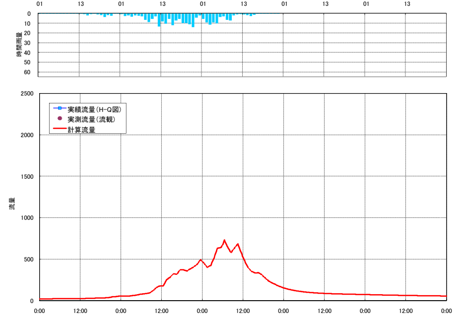
流出計算結果 平成13年9月洪水 上久屋 (片品川)
