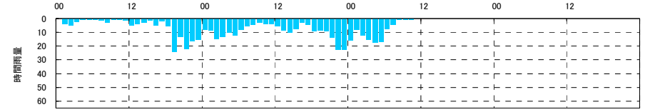
流出計算結果 平成19年9月洪水 岩鼻（烏川）
