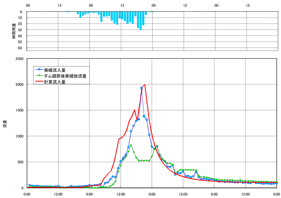
流出計算結果 平成11年8月洪水 下久保ダム（神流川）
