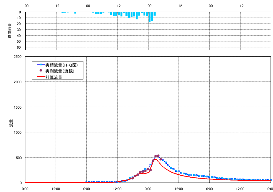
流出計算結果 平成14年7月洪水 万場（神流川）
