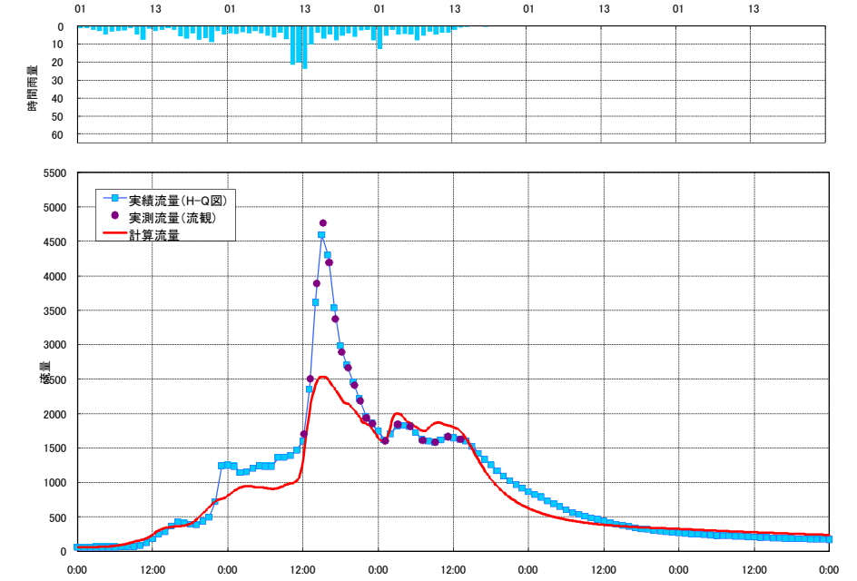
流出計算結果 平成13年9月洪水 八斗島 (利根川)
