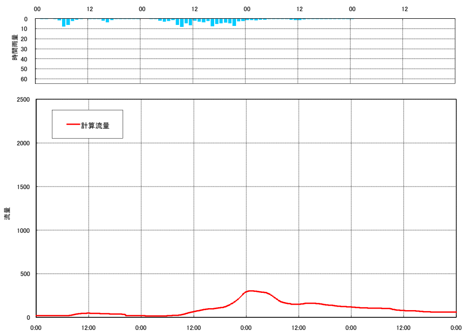
流出計算結果 平成11年8月洪水 上久屋 (片品川)
