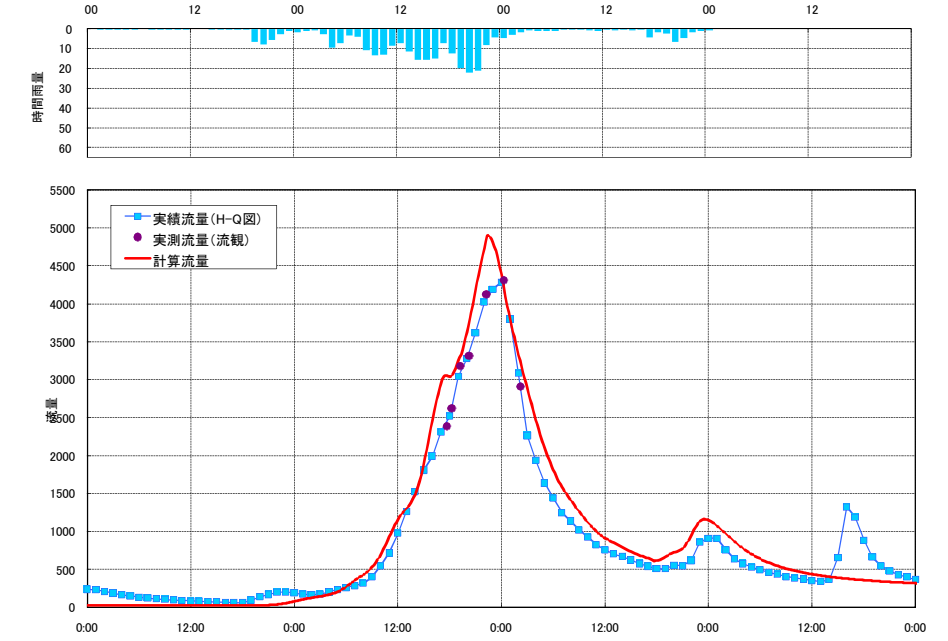
流出計算結果 平成11年8月洪水 八斗島 (利根川)
