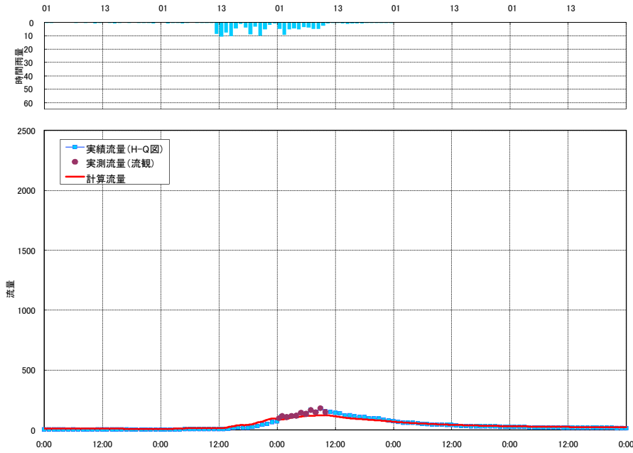
流出計算結果 平成13年9月洪水 藪原ダム (片品川)
