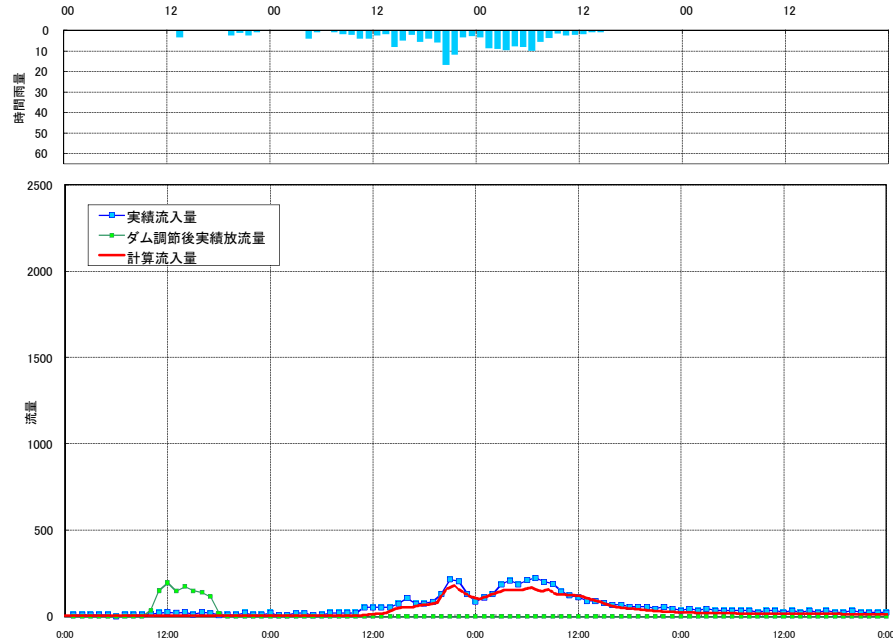
流出計算結果 平成14年7月洪水 藤原ダム (利根川)
