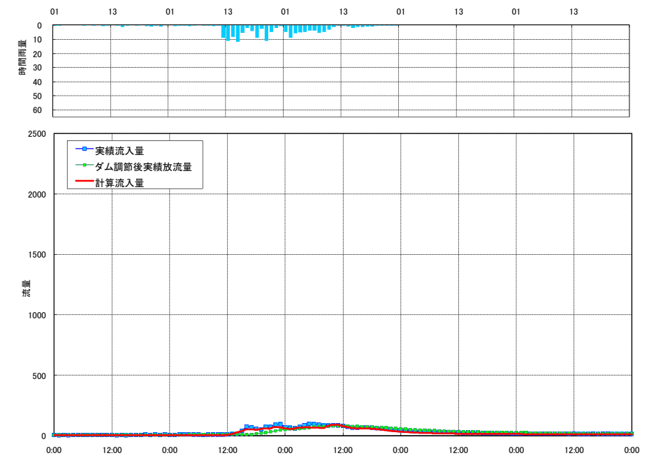
流出計算結果 平成13年9月洪水 相俣ダム (赤谷川)
