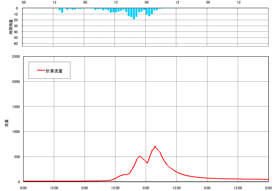
流出計算結果 平成14年7月洪水 上久屋 (片品川)
