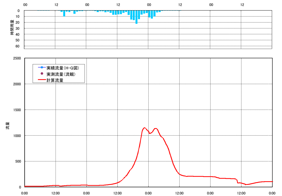
流出計算結果 平成14年7月洪水 上久屋 (片品川)
