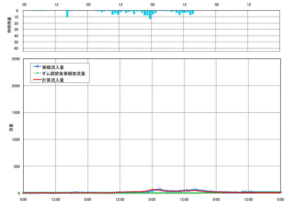
流出計算結果 平成11年8月洪水 相俣ダム (赤谷川)
