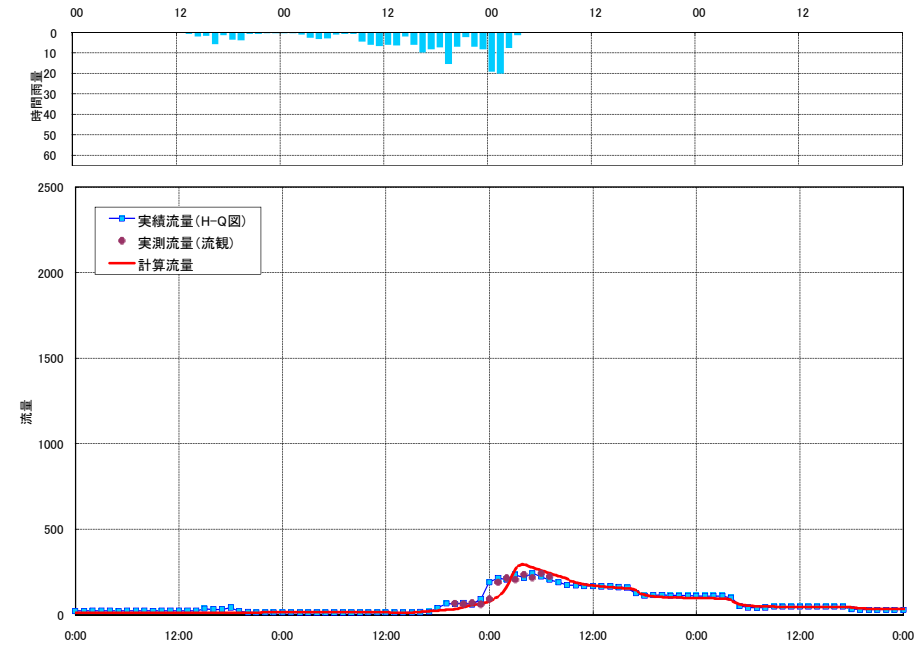
流出計算結果 平成14年7月洪水 若泉 (神流川)
