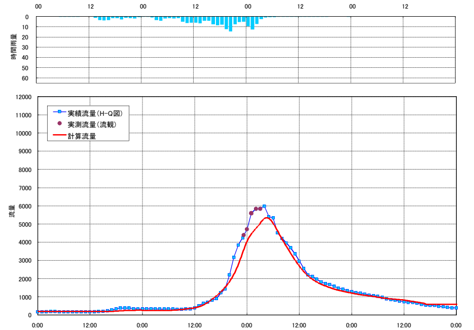
流出計算結果 平成14年7月洪水 八斗島 (利根川)
