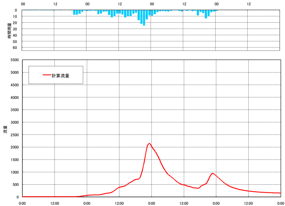
流出計算結果 平成11年8月洪水 万場（神流川）
