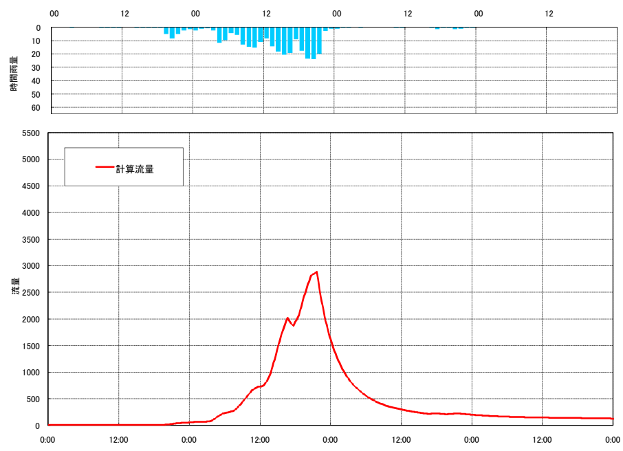
流出計算結果 平成11年8月洪水 下久保ダム（神流川）
