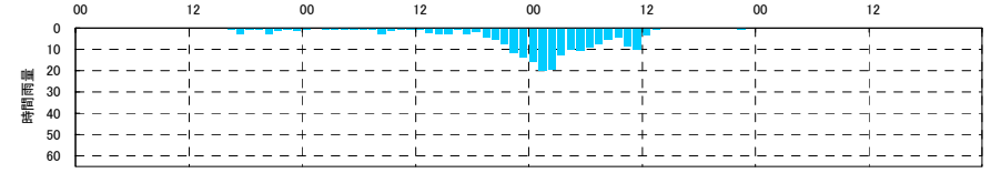
流出計算結果 平成19年9月洪水 千鳥 (片品川)
