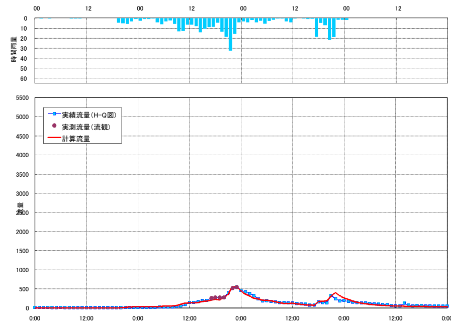
流出計算結果 平成11年8月洪水 安中 (碓氷川)
