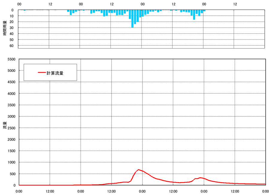
流出計算結果 平成11年8月洪水 上里見 (烏川)
