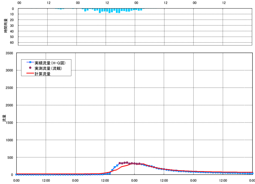
流出計算結果 平成14年7月洪水 上里見 (烏川)
