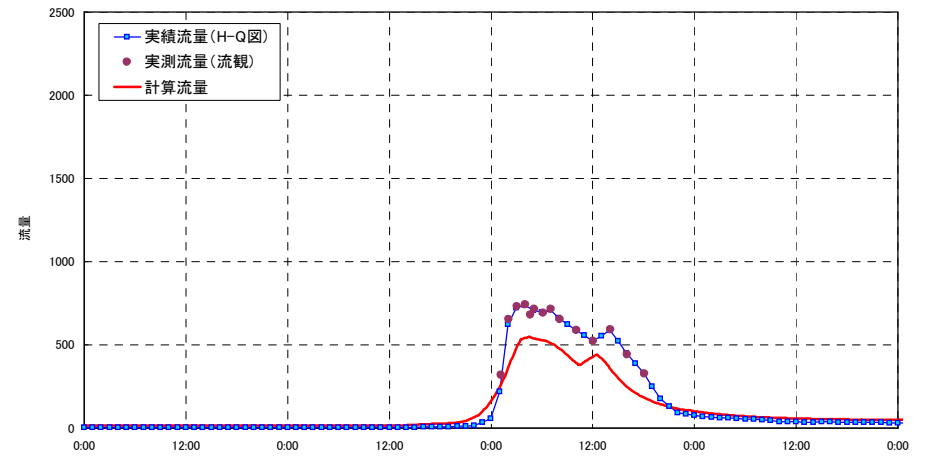
流出計算結果 平成19年9月洪水 上久屋 (片品川)
