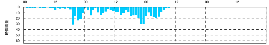
流出計算結果 平成19年9月洪水 岩井（鑛川）
