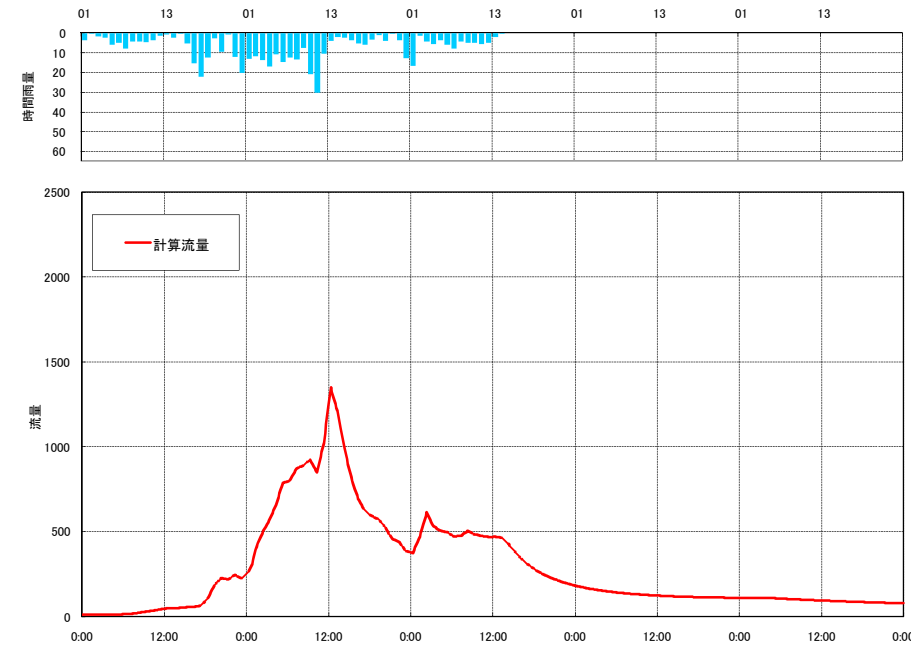
流出計算結果 平成13年9月洪水 万場（神流川）
