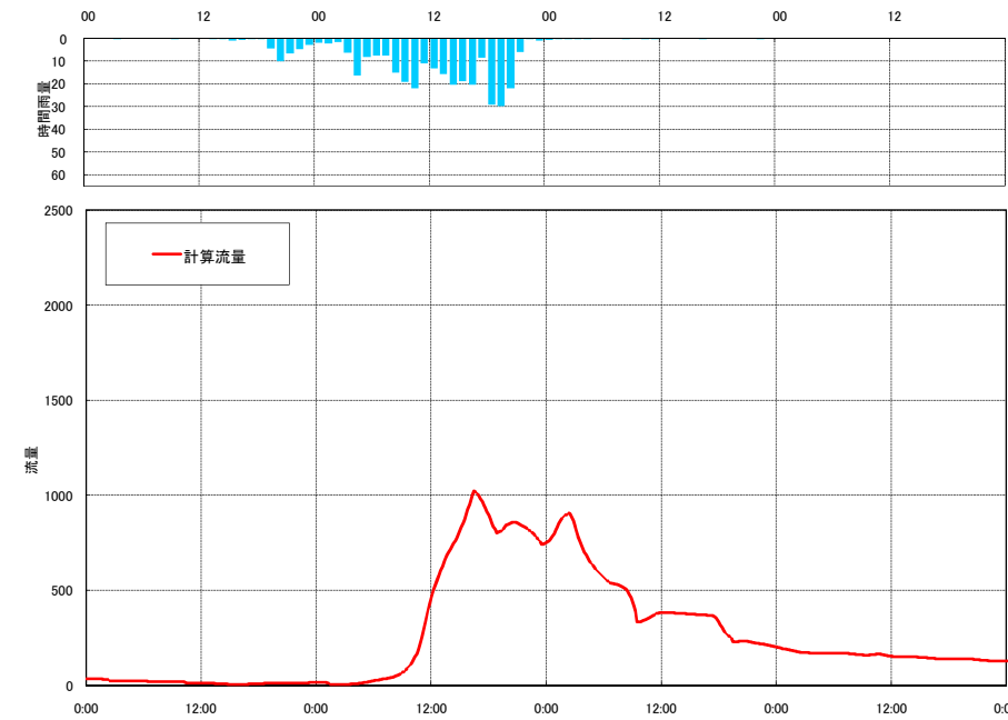
流出計算結果 平成11年8月洪水 若泉 (神流川)
