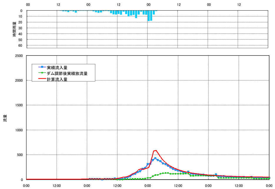
流出計算結果 平成14年7月洪水 下久保ダム（神流川）
