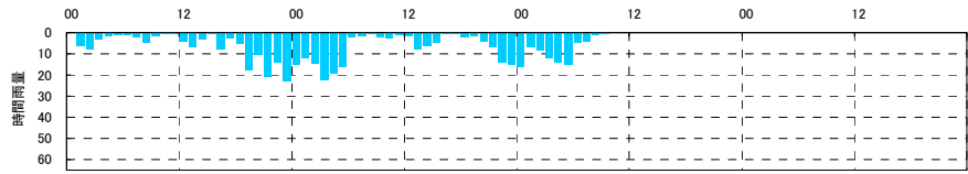
流出計算結果 平成19年9月洪水 高松（烏川）
