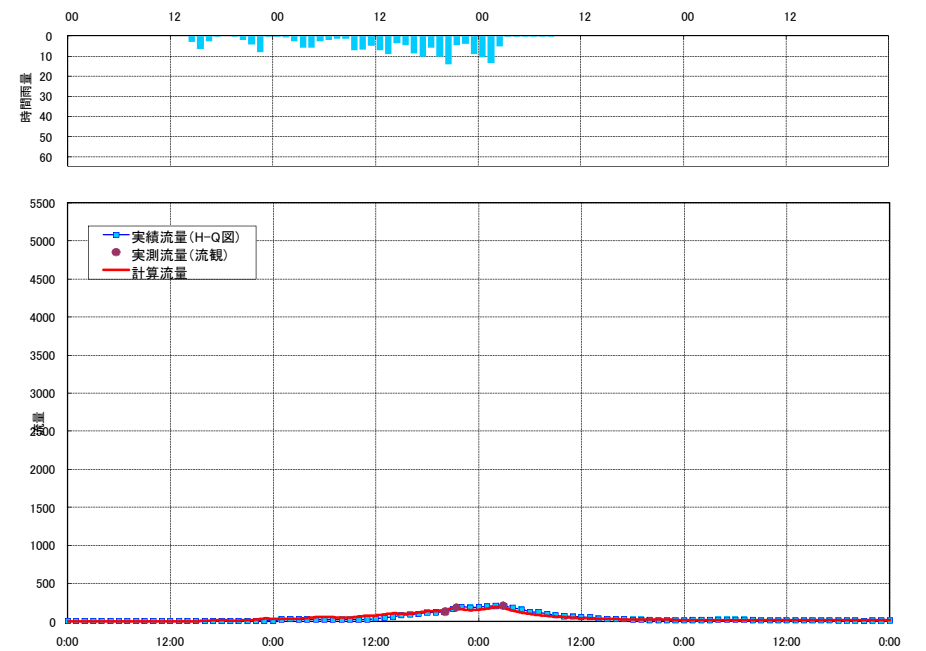
流出計算結果 平成14年7月洪水 安中 (碓氷川)
