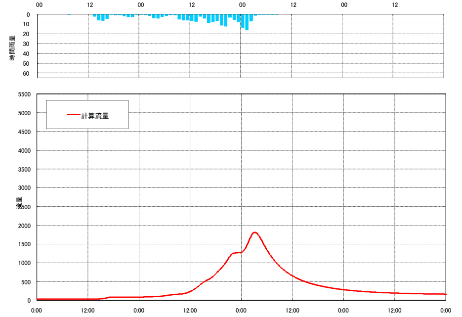
流出計算結果 平成14年7月洪水 八斗島 (利根川)
