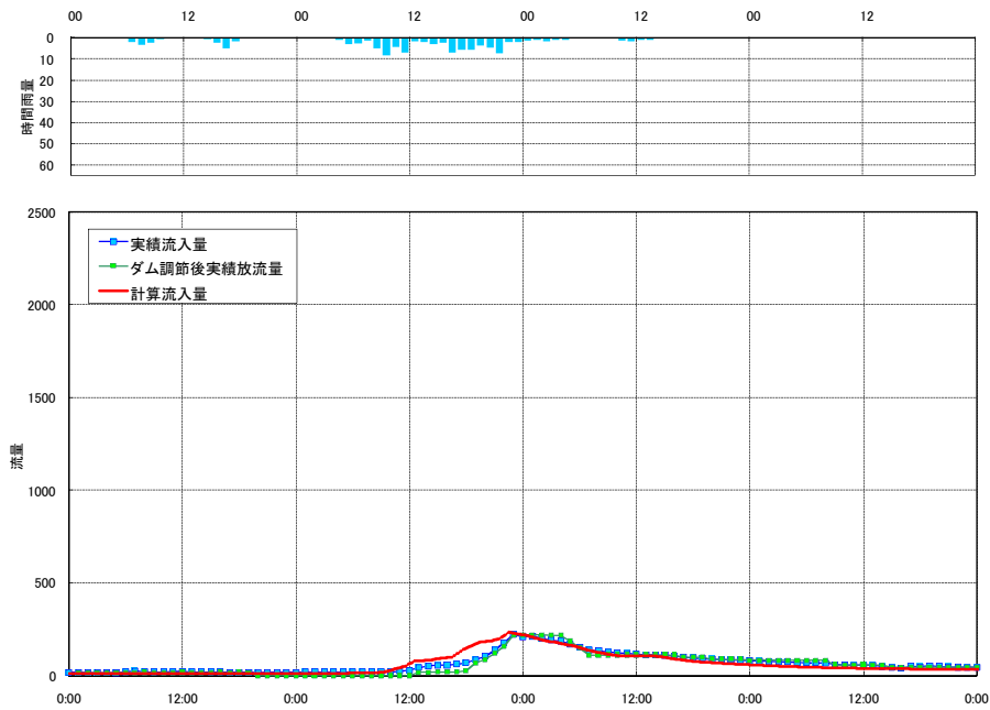
流出計算結果 平成11年8月洪水 藪原ダム (片品川)
