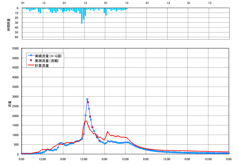
流出計算結果 平成13年9月洪水 下久保ダム（神流川）
