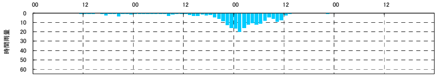
流出計算結果 平成19年9月洪水 上久屋 (片品川)
