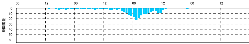
流出計算結果 平成19年9月洪水 藪原ダム (片品川)
