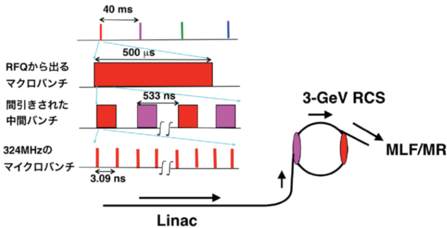
Fig. 17 チョッパーによる中間バンチ形成 (2018/10/02)
