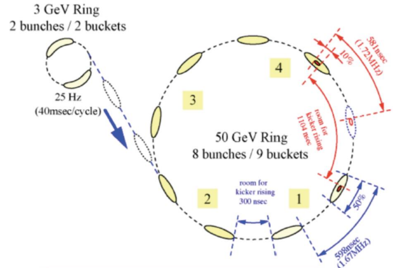
Fig. 19 RCS と MR のビームバンチ
